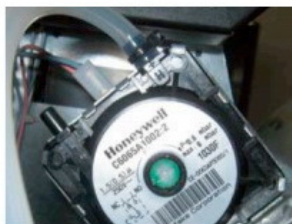
Control de la presión de aspiración de las cámaras internas de la estufa.
